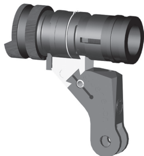
Bild 13: Universalkornträger zu Stgw 57 (Normalmontage), diverse Fabrikate
