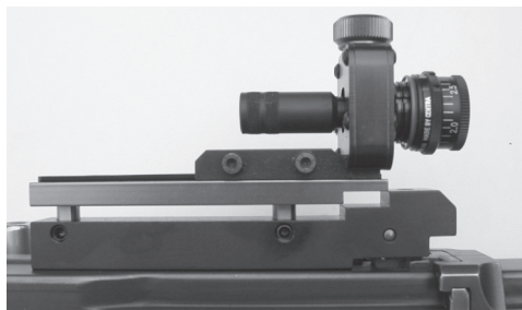
Bild 16: Diopterträger zu Stgw 57 zur Aufnahme schussfester Diopter, diverse Fabrikate
