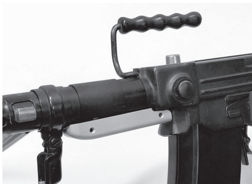
Bild 21: Handschutz zu Stgw 57
