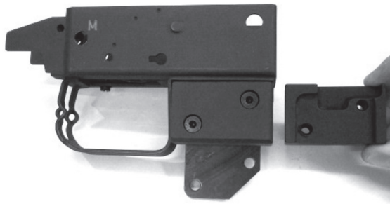
Bild 19: Griffadapter zu Stgw 57
